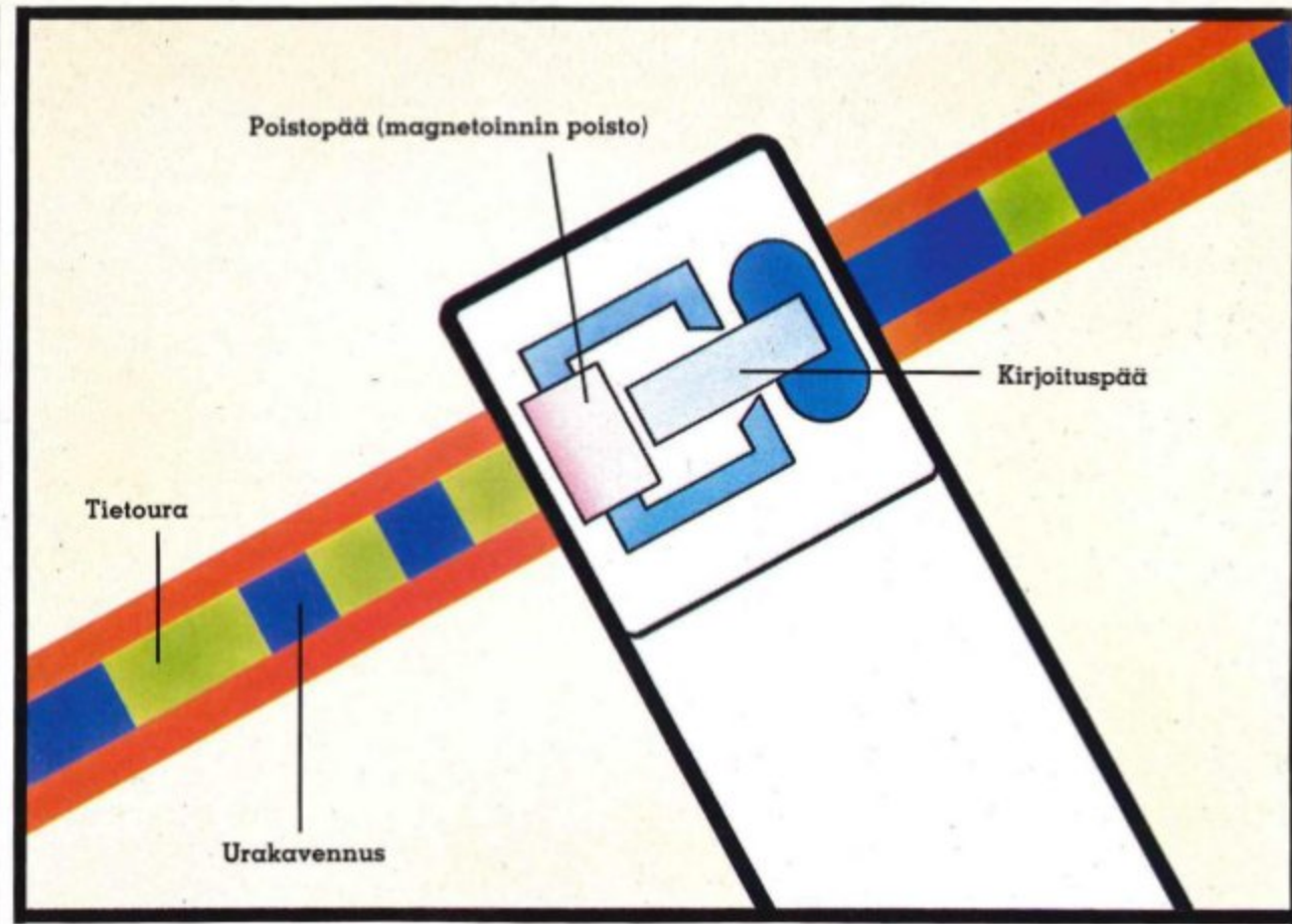
Näin saadaan aikaan tietoura: Kirjoitus- ja lukupää välittää tiedot elektromagneettisina impulsseina. Pyyhinpää kaventaa tietouraa järjestämällä sen oikealle ja vasemmalle puolelle yhtenäiset magneettikentät.
