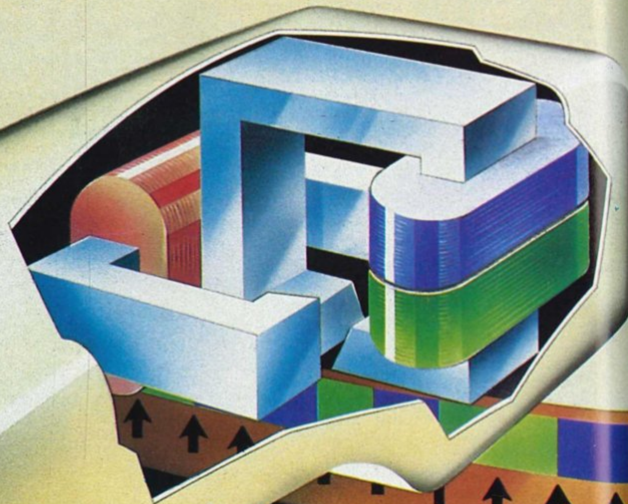
Kaksi ferriittikappaletta kirjoitus- ja lukupäässä magnetoivat kelojen (vihreä, sininen, punainen) avulla tietouran levykkeelle. Suurennoa seuraavalla sivulla olevasta nuolella merkitystä kohdasta.
