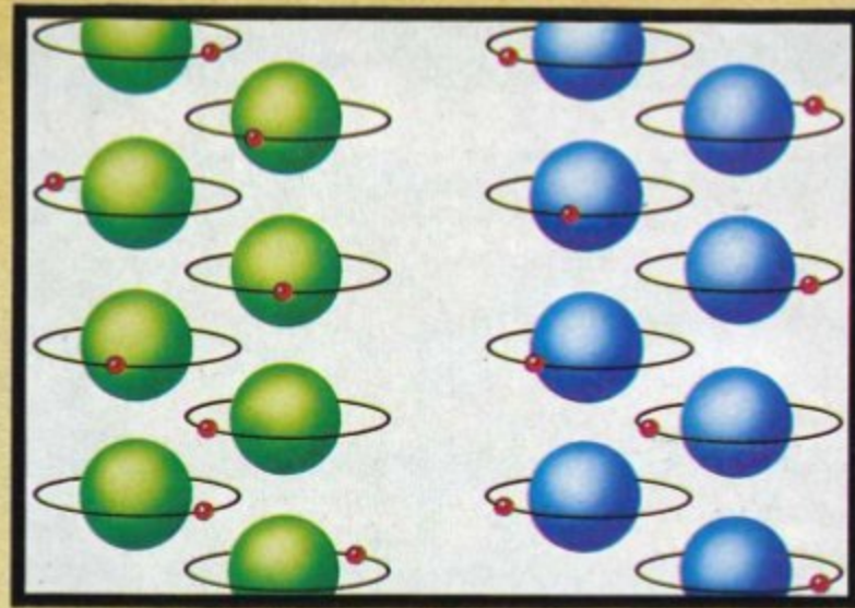
Tämä kuva kertoo, miten magneettisuus ilmiönä voidaan selittää yksinkertaisesti: Elektronien (esimerkiksi raudan elektronien) kiertosuunta atomiytimen ympäri voidaan säädellä. Niiden kiertosuunta riippuu magnetointitavasta. Jos magnetointiin käytetään pohjoisnapaa (siniset atomit), niin kiertosuunta on päinvastainen kuin etelänavan kanssa magnetoitaessa (vihreät atomit).
