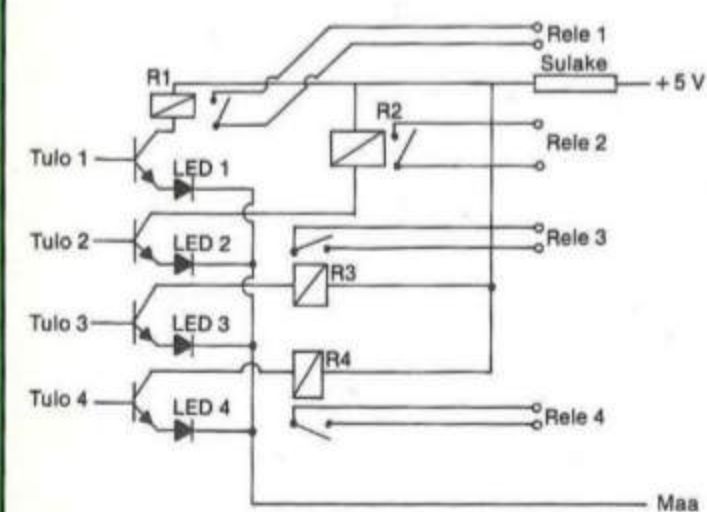
Kytkentäkaavio
