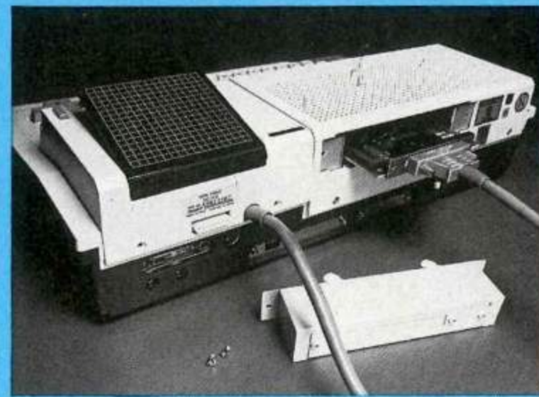
MZ Disk -levyasema asetetaan kasettinauhuriin tilalle ja liitetään kaapelilla laajennusporttiin työnnettynä sovittynsikköön.
