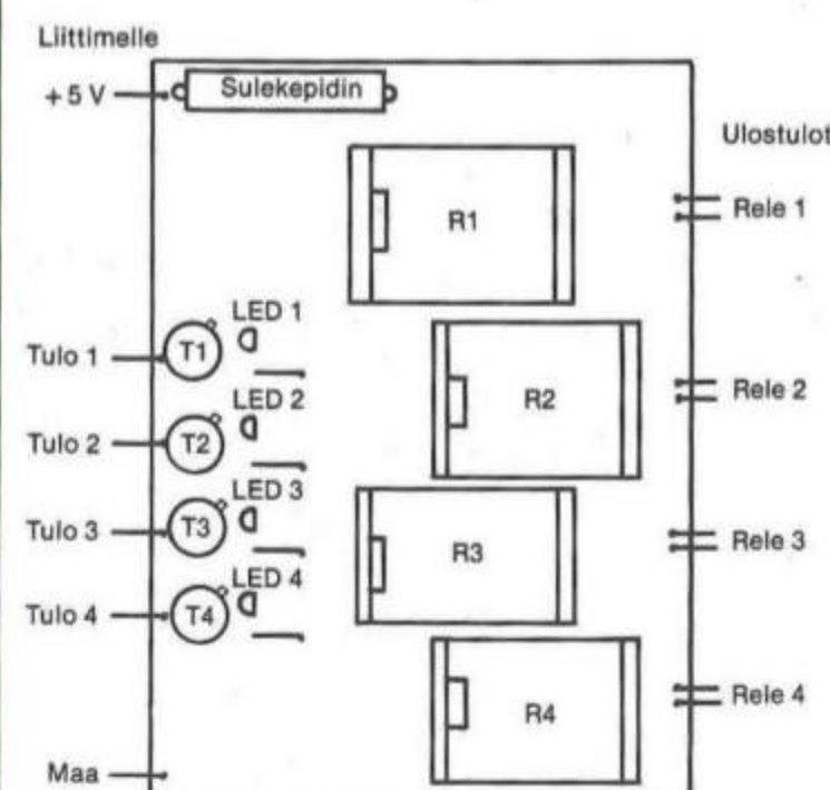
Komponenttisijoittelu ylhäältä katsottuna
