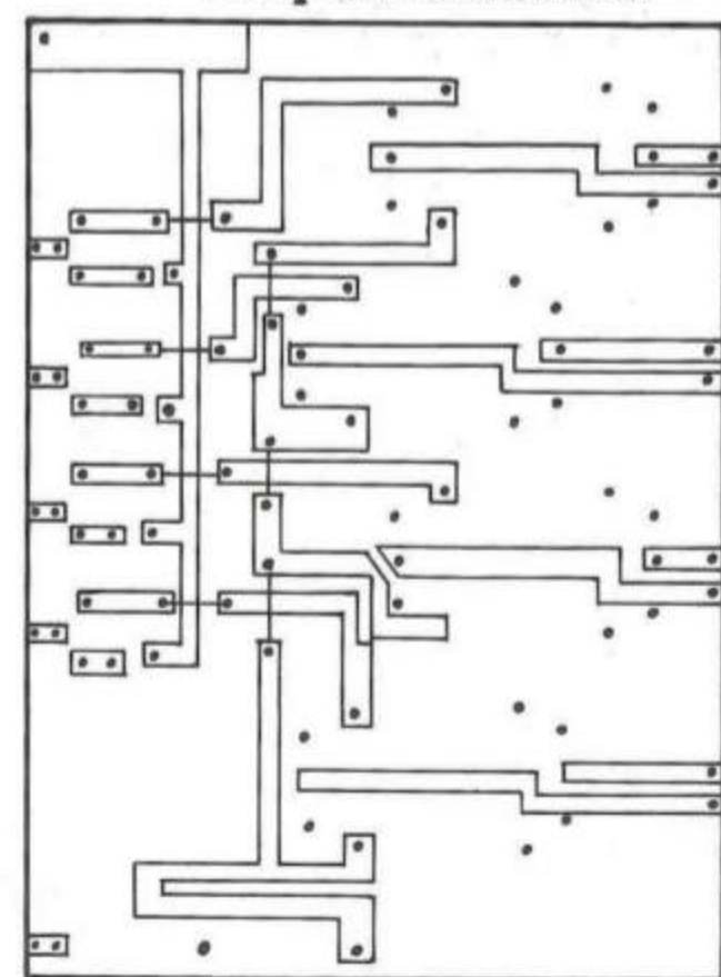
Releohjaimen piirilevy altapäin katsottuna
