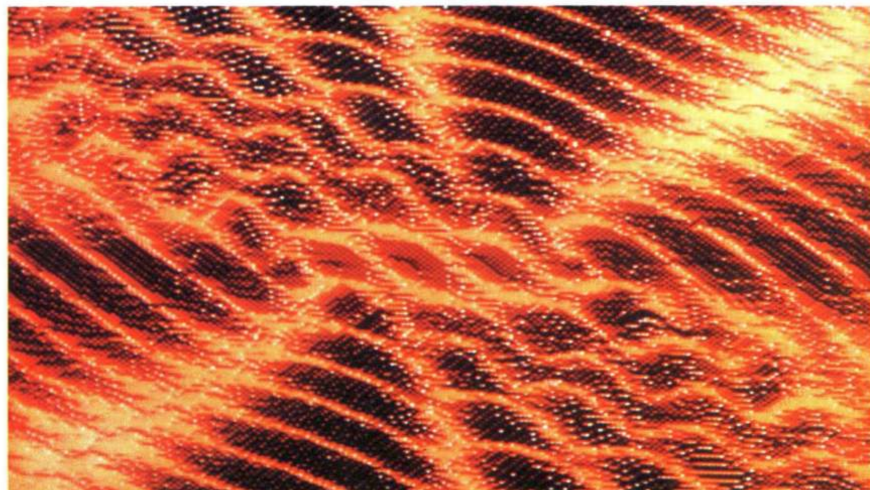
Kahden samantaajuisen värähtelylähteen interferenssi. Värähtelijät ovat kuvan keskellä vierekkäin (paikallistaminen vaikeaa).
