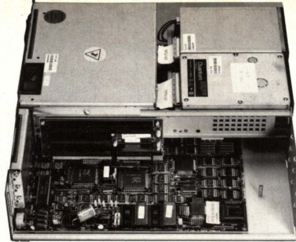
Citizenin emokortti peittää melkein koko pohjan. Lisäkortteja voi kiinnittää vaakatasoon emokortin yläpuolelle.
